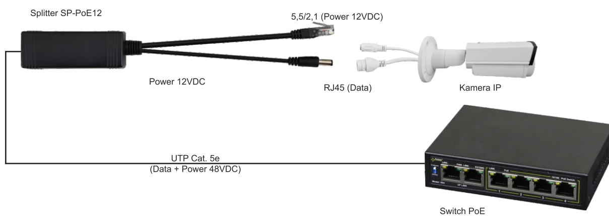
Rys. 2. Przykład podłączenia ze Switch'em PoE.
