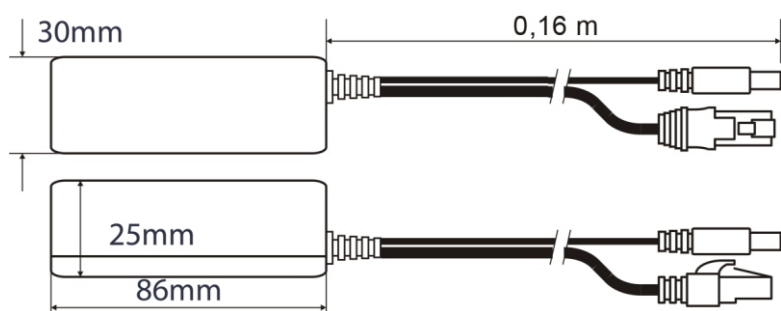
Rys. 1. Widok mechaniczny
